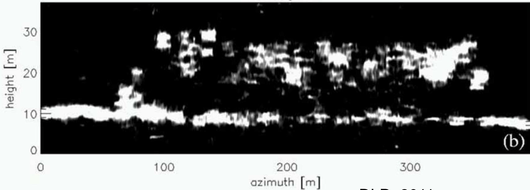
Tomogram
